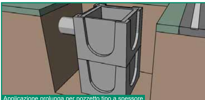
Applicazione prolunga per pozzetto tipo a spessore
