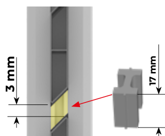
Ⓒ Distanziatori per Occultante Parziale
