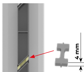
Ⓓ Distanziatori per Occultante Totale
