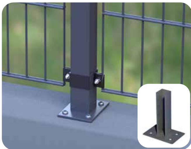
Per la posa su muretto con supporto
