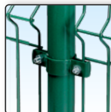
Palo Tubolare Ø 48 mm con collari in acciaio Vedi a pag. 12/13
