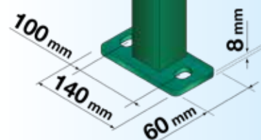
Piastra saldata al palo QUADRO
