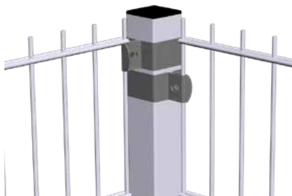
Collare semplice in acciaio
