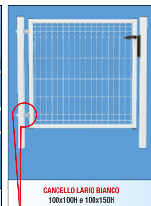
Nuova cerniera "Pro"
